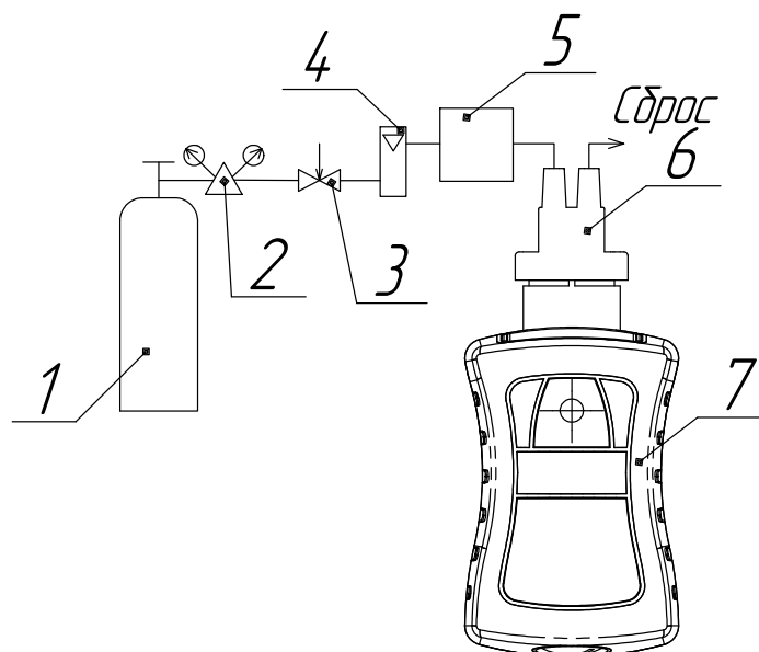
а) газоанализаторы АНКAT-7631Микро-СО, АНКАТ-7631Микро-О 2 , АНКАТ-7631Микро-НН 3
